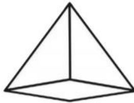
pyramid
