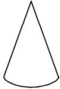
cone
